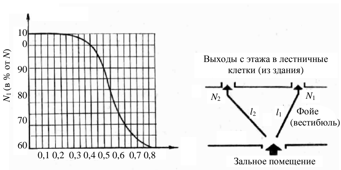
Рис. П5.5., а. Число зрителей и выбор выхода при эвакуации в две лестничные клетки либо в две открытые лестницы или в два выхода из здания: N – общее количество эвакуирующихся; N_1 – число эвакуирующихся через ближний выход; N_2 – число эвакуирующихся через дальний выход; l_1 – длина пути до ближнего выхода; l_2 – длина пути до дальнего выхода
