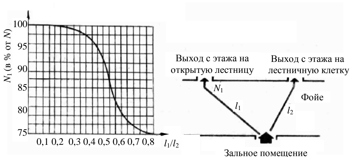
Рис. П5.5., б. Число зрителей эвакуирующихся по открытой лестнице: N – общее количество эвакуирующихся; N_1 – число эвакуирующихся по открытой лестнице; l_1 – длина пути до открытой лестнице; l_2 – длина пути до выхода в лестничную клетку
